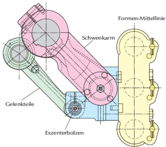
Stationsgehäuse
